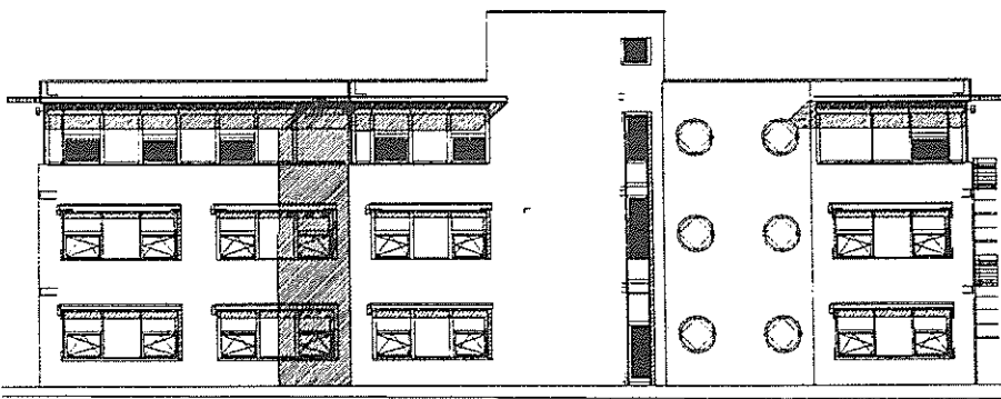
Ansicht Süd
