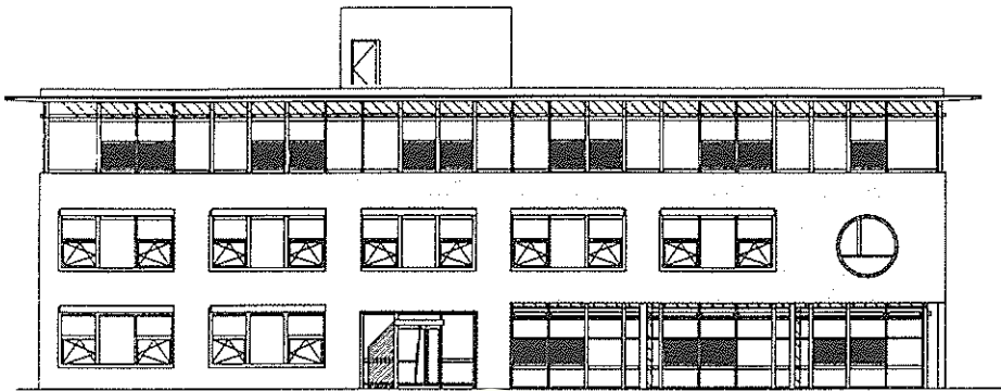
Ansicht Nord
